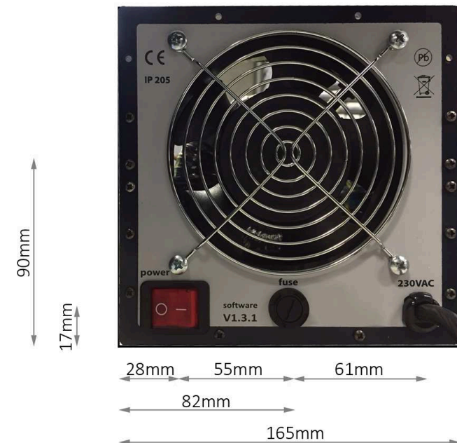
Achteraanzicht
