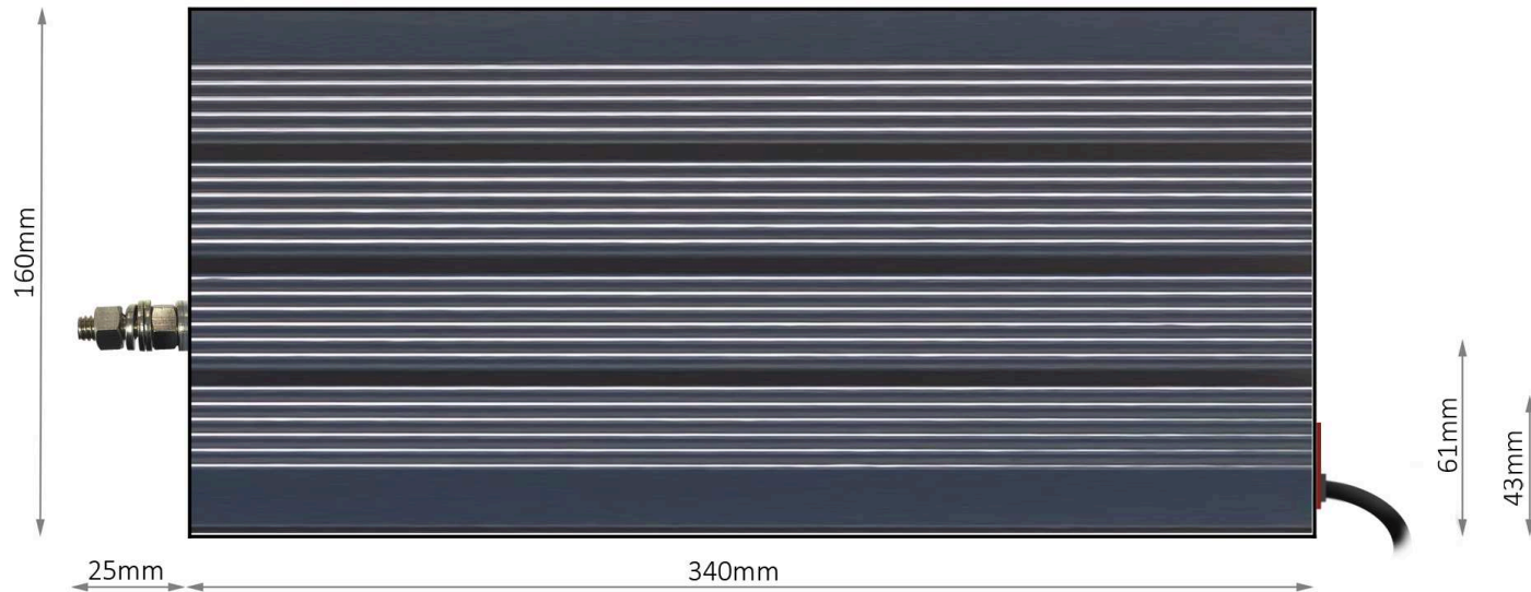
Rechterzijaanzicht
